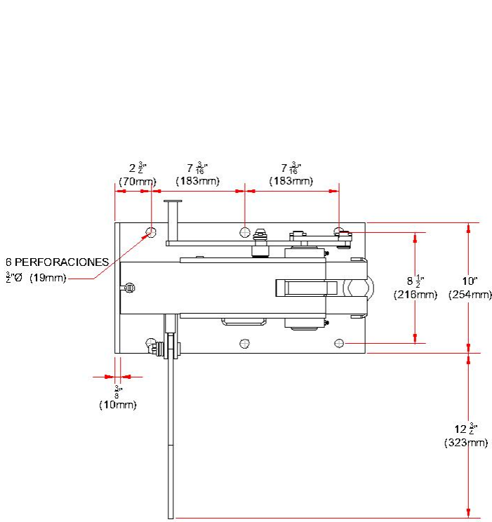
Vista Superior
